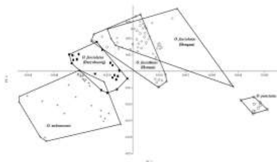
شکل ۲- نمودار تجزیه به مؤلفه‌های اصلی (PCA) شکل بدن جمعیت‌های بلنی ماهیان مورد مطالعه
