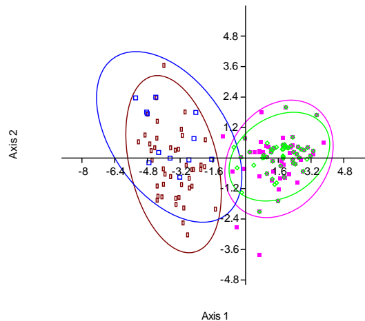
شکل ۵- پراکنش ایستگاه‌ها در نمودار CVA با استفاده از محور ۱ و ۲ (اتولیت چپ)
