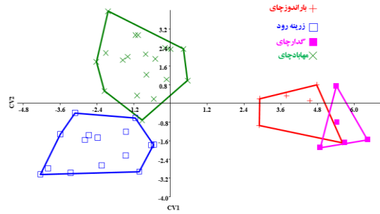
شکل ۴- نمودار تجزیه همبستگی کانونی شکل بدن جمعیت‌های مورد مطالعه جویبار ماهی السا ( O. elsae ) با درجه صحیح کلاس بندی شده ۹۶/۱۵ در حوضه دریاچه ارومیه
