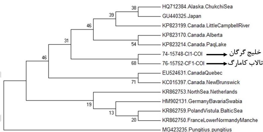
شکل ۲- درخت تبارشناسی به روش پیوند همجواری (NJ) ماهی سه خار (G. aculeatus) با برون گونه Pungitius pungitius
