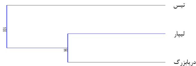
شکل ۷- نمودار تحلیل خوشه‌ای شکل بدن سه جمعیت (تیس، لیپار و دریابزرگ) گونه I.spilotus
