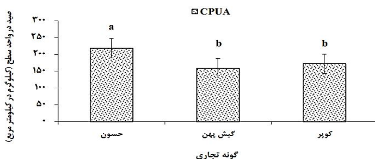
شکل ۲- مقدار CPUE سه گونه حسون معمولی ( S. tumbil )، گیش پهن ( C. talamparoides ) و کوپر ( A. spinifer )، در تورهای ترال کف در آبهای استان بوشهر در سال ۱۳۹۲
