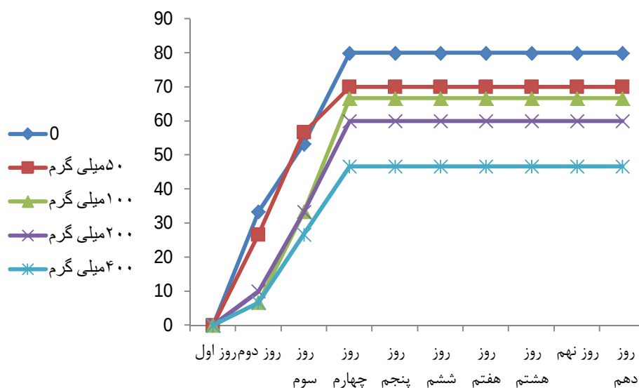
شکل ۱- درصد تلفات تجمعی ماهی قزل آلای رنگین کمان ( O. mykiss ) تغذیه شده با سطوح مختلف جلبک دریایی سارگاسوم انگستیفلیوم در برابر باکتری یرسینیا راکری
