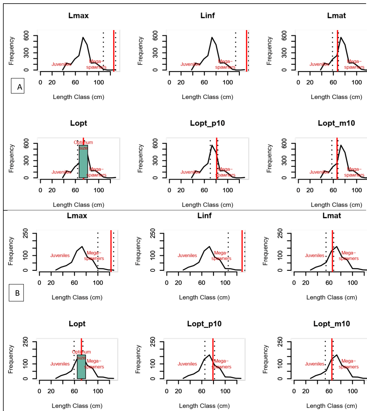
شکل ۵: طول حداکثر ( L_{\max} )، طول بی نهایت ( L_{\infty} )، طول بلوغ ( L_{\text{mat}} )، طول بهینه ( L_{\text{opt}} )، ده درصد حد بالایی طول بهینه ( L_{\text{opt\_p10}} ) و ده درصد حد پایینی طول بهینه ( L_{\text{opt\_m10}} ) ماهی هورور طی سال های ۱۳۷۳ (A) و ۱۴۰۳ (B) در آب های شمالی دریای عمان (استان سیستان و بلوچستان)
