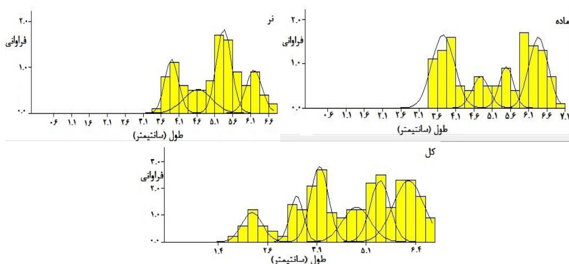
شکل ۸- نمودارهای توزیع فراوانی طولی گروه‌های همزاد جداسازی شده ماهی سه خارده جنوب شرق دریای خزر
