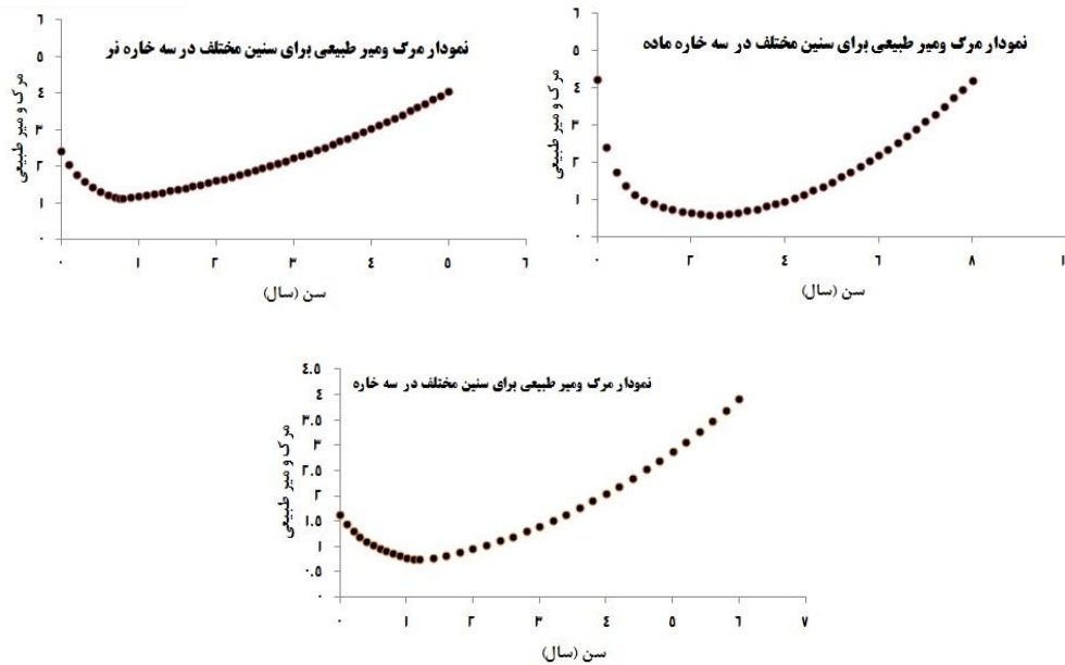
شکل ۶- میزان مرکب و میر طبیعی برآورده به روش چن و واتابه برای ماهی سه خارده در سنین مختلف
