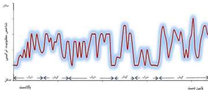
شکل ۱۰- توزیع مطلوبیت زیستگاهی گونه سیاه‌ماهی در بازه‌های رودخانه زرین‌گل
