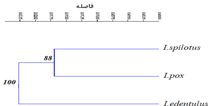
شکل ۴- نمودار تحلیل خوشه‌ای شکل بدن سه گونه مورد مطالعه
