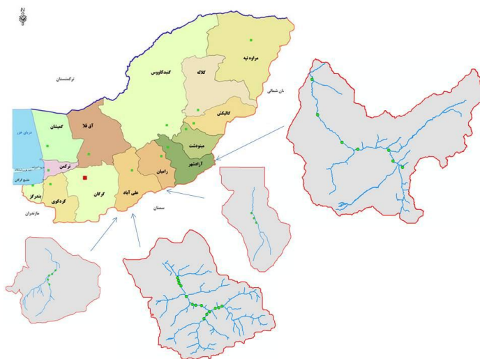
شکل ۱- موقعیت مکانی هر یک از حوضه های آبخیز در استان گلستان
