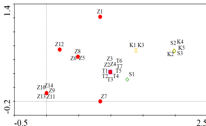
شکل ۲ ب- نمودار پراکندگی ایستگاه های نمونه برداری براساس داده های حضور و عدم حضور در آنالیز DCA علامت دایره های قرمز نهر زیرین گل، مربع آبی نهر تیل آباد، مستطیل نهر کبودوال و لوزی نهر شیرآباد.
