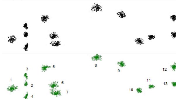
شکل ۱- میزان جابجایی و تغییرات در موقعیت لندمارک‌ها نسبت به شکل میانگین نمونه‌های مورد مطالعه سیاه‌ماهی خال‌دار مند ( C. manduca )
