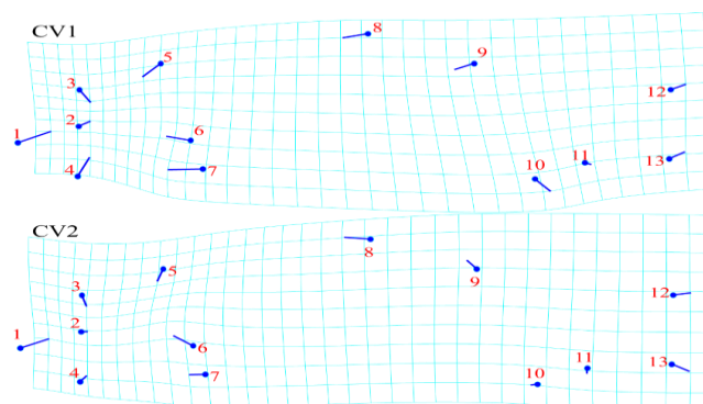
شکل ۶- تغییرات شکل بدنی نمونه‌های سیاه‌ماهی خال‌دار مند ( C. mandica ) در جهت هریک محورهای CV_1 و CV_2
