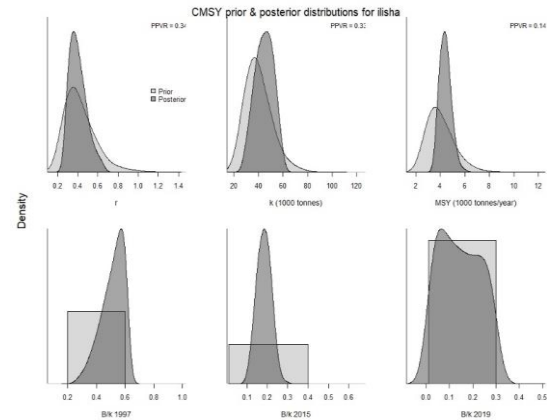
شکل ۳- نتایج مربوط به مدل صید-حداکثر محصول پایدار (CMSY) برای ماهی صبور ( T. ilisha ) در آب‌های جنوبی ایران از سال ۱۳۷۶-۱۳۹۸.
