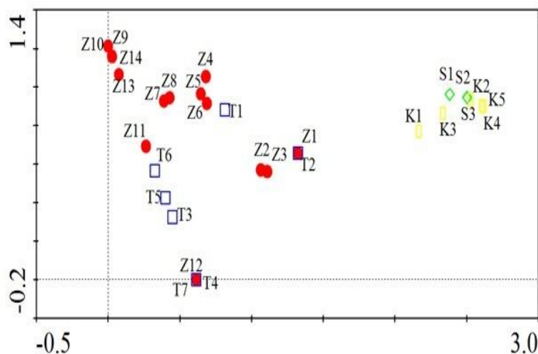
شکل ۳ ب- نمودار پراکندگی ایستگاه‌های نمونه‌برداری براساس داده‌های حضور و عدم حضور در آنالیز DCA علامت دایره‌ای قرمز زرين گل، مربع آبی نهر تیل آباد، مستطیل نهر کبودوال و لوزی نهر شیرآباد.
