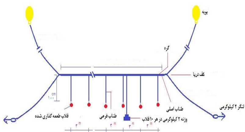
شکل ۲- طرح کلی رشته قلاب طویل مورد استفاده در این تحقیق
