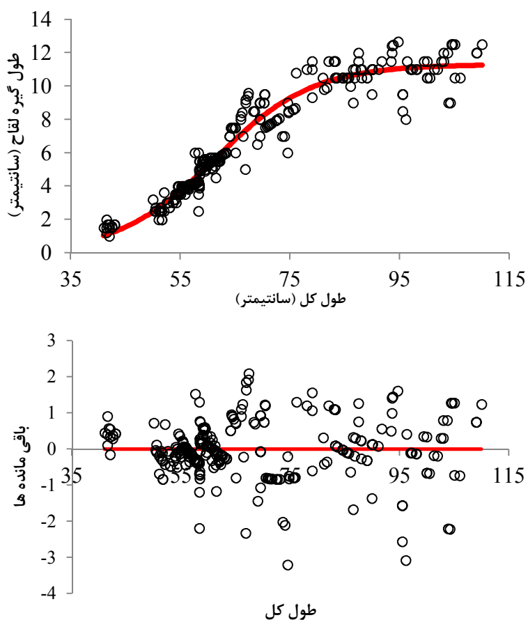
شکل ۴- ارتباط بین طول کلاسیک و طول کل در کوسه چانه سفید ( C. dussumieri ) و آنالیز باقی مانده‌ها
