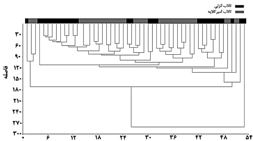
شکل ۵- دندروگرام UPGMA صفات ريختی بر اساس فاصله اقليدسی اردك ماهی تالاب‌های انزلی و امير كلايه
