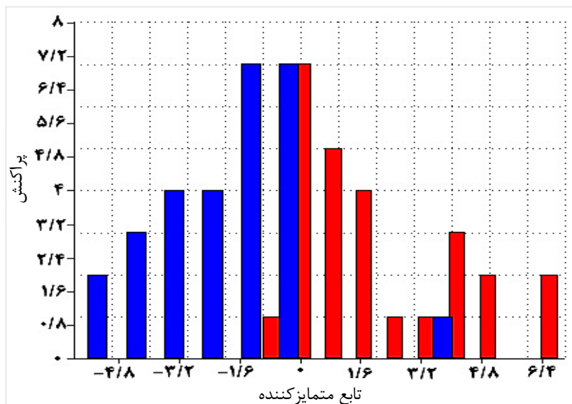
شکل ۴- پراكنش افراد بر اساس مقادير تابع متمايزكننده ۱ و ۲ ريختی اردك ماهی تالاب‌های انزلی و امير كلايه
