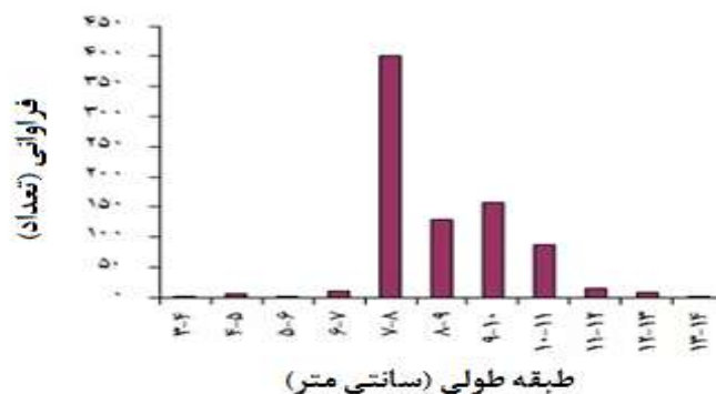
شکل ۲- فراوانی طولی چغوک نقره‌ای معمولی ( G. omya ) در خوریات ذخیره‌گاه زیست‌کره حرا - استان هرمزگان (۱۳۹۵-۱۳۹۶)
