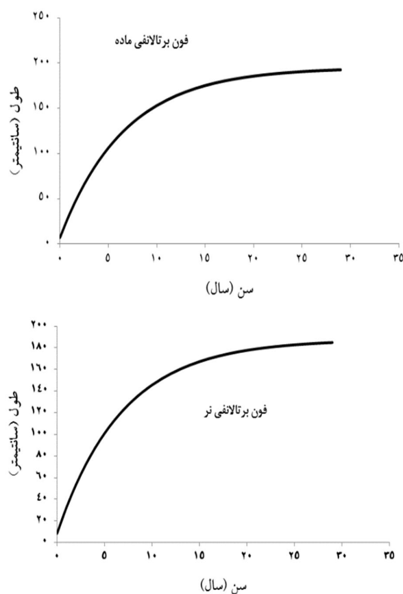
شکل ۵- رابطه طول- سن جنس نر و ماده ماهی ازون برون ( A. stellatus ) به روش فون پرتالانفی در آب‌های حوضه جنوبی دریای خزر
