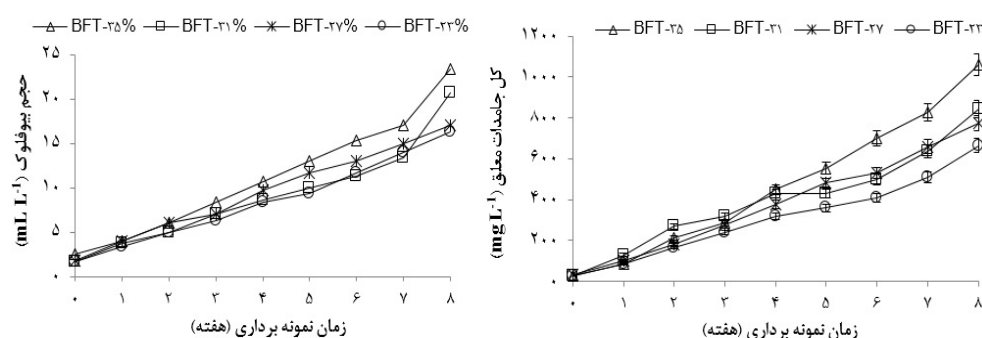
شکل ۱- تغییرات BFV و TSS در چهار تیمار بررسی تعیین سطح مناسب پروتئین جیره غذایی بچه‌ماهی کپور معمولی ( C. carpio ) بر پایه فناوری بیوفلاک طی ۸ هفته دوره آزمایشی. هر مقدار نشان دهنده میانگین \pm انحراف معیار است ( n=3 ).
