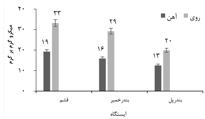
شکل ۵- مقایسه عناصر آهن و روی در عضله ماهی شوروت ( S. Sihama ) در مناطق قشم، بندر خمیر و بندر پل در فصل تابستان
