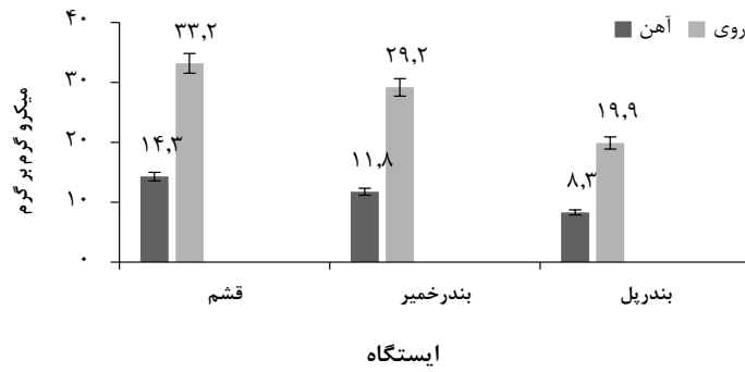
شکل ۳: مقایسه عناصر آهن و روی در عضله ماهی شوروت ( S. Sihama ) در مناطق قشم، بندر خمیر و بندر پل در فصل زمستان
