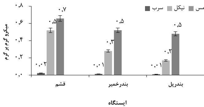
شکل ۴- مقایسه عناصر نیکل، سرب و مس در عضله ماهی شوروت ( S. Sihama ) در مناطق قشم، بندر خمیر و بندر پل در فصل تابستان
