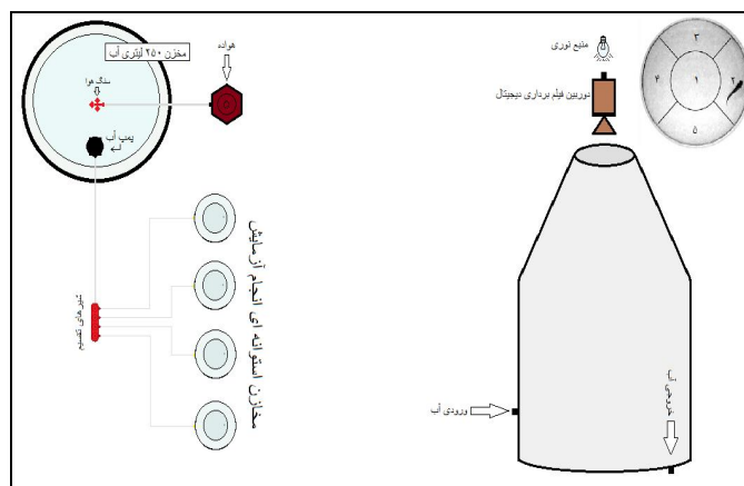
شکل ۱- تصویر شماتیک محیط آزمایش به همراه اجزای تشکیل‌دهنده آن و سیستم‌های فیلم‌برداری و جمع‌آوری اطلاعات بررسی ارزیابی پاسخ‌های رفتاری بچه‌ماهی قزل‌آلای رنگین‌کمان ( O. mykiss ) در مواجهه با تغییرات محیطی
