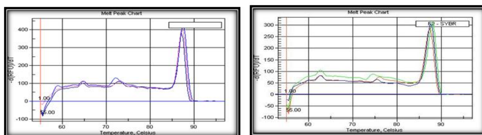
شکل ۲- منحنی ذوب ترسیم شده از غلظت‌های سریالی برای آغازگر \beta -actin (شکل راست) و منحنی ذوب ترسیم شده از غلظت‌های سریالی برای آغازگر P450 (شکل چپ).
