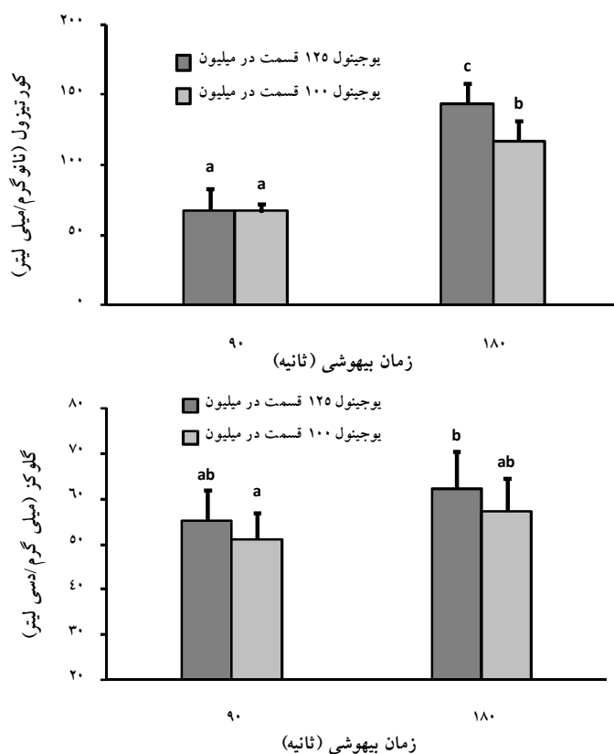
شکل ۲- سطوح کورتیزول (شکل بالا) و گلوکز (شکل پایین) سرم ماهی قرمز پس از ۹۰ و ۱۸۰ ثانیه بیهوشی توسط ۱۰۰ و ۱۲۵ قسمت در میلیون یوجینول. حروف متفاوت نشان دهنده اختلاف معنی‌دار هستند.
